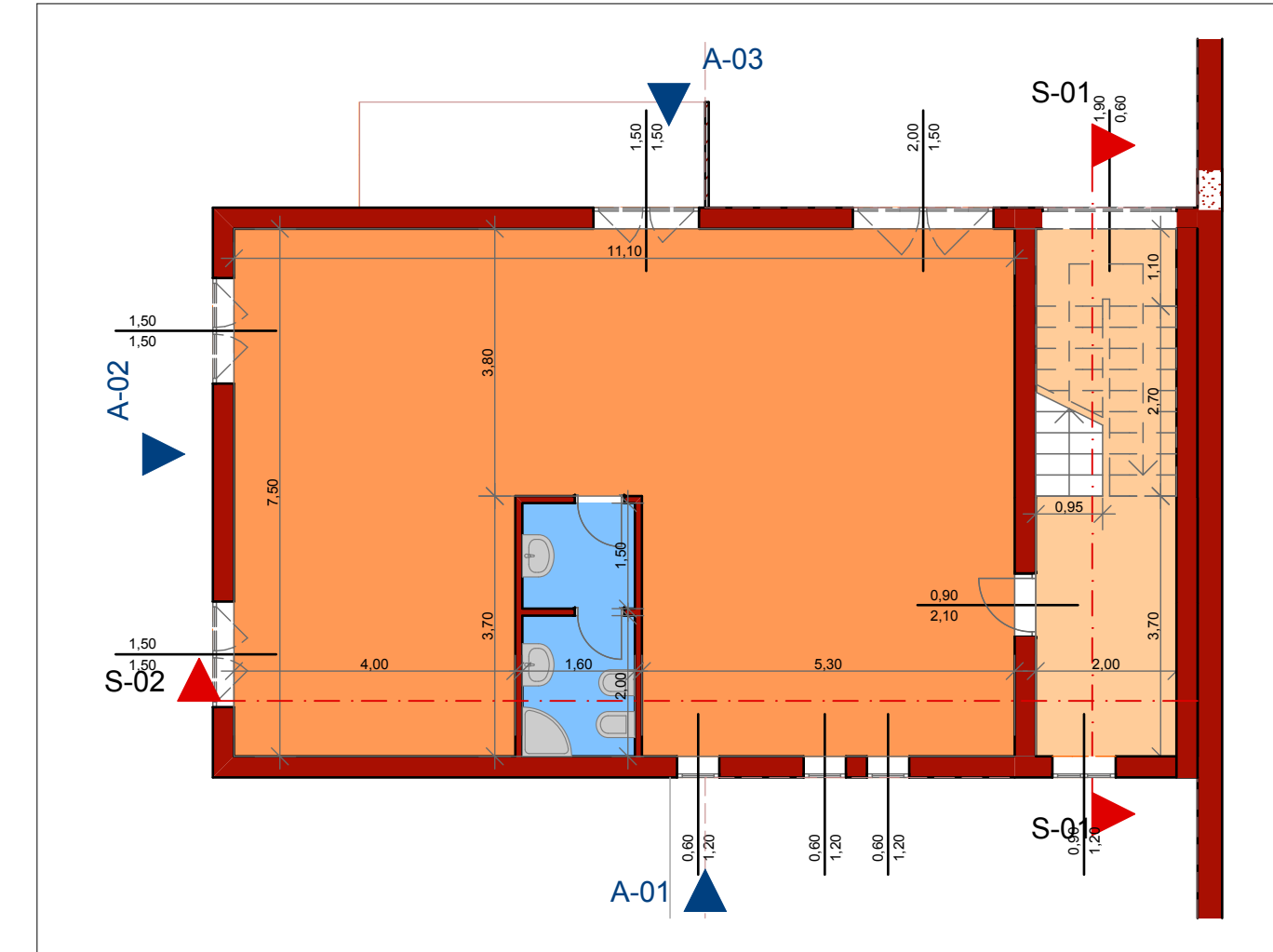
1.2. PIANO PRIMO - SECONDO 1:100
