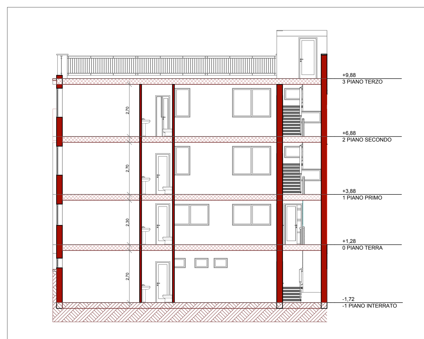
S-02 SEZIONE 1:100
