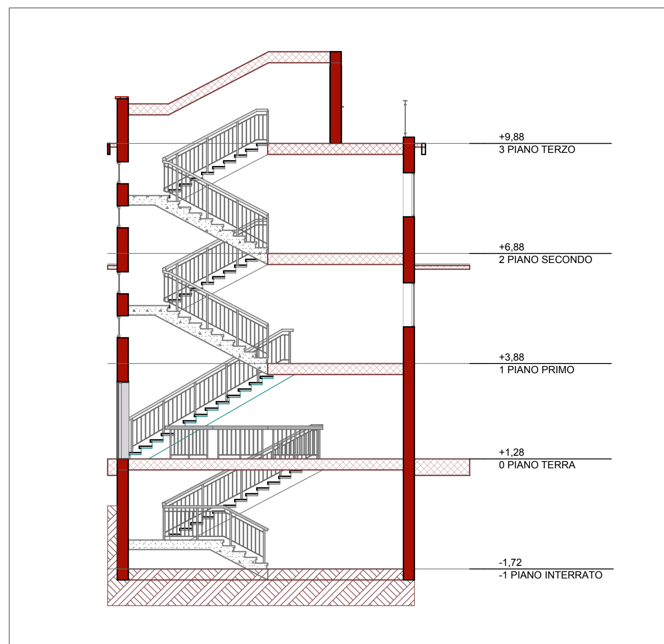
S-01 SEZIONE 1:100
