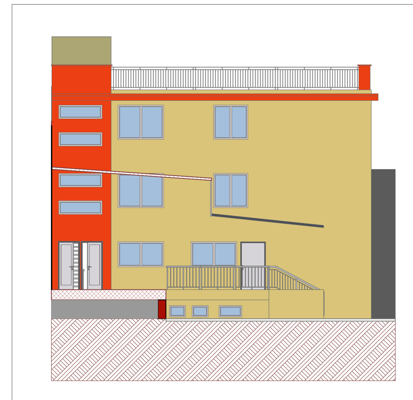
A-03 PROSPETTO 1:100
