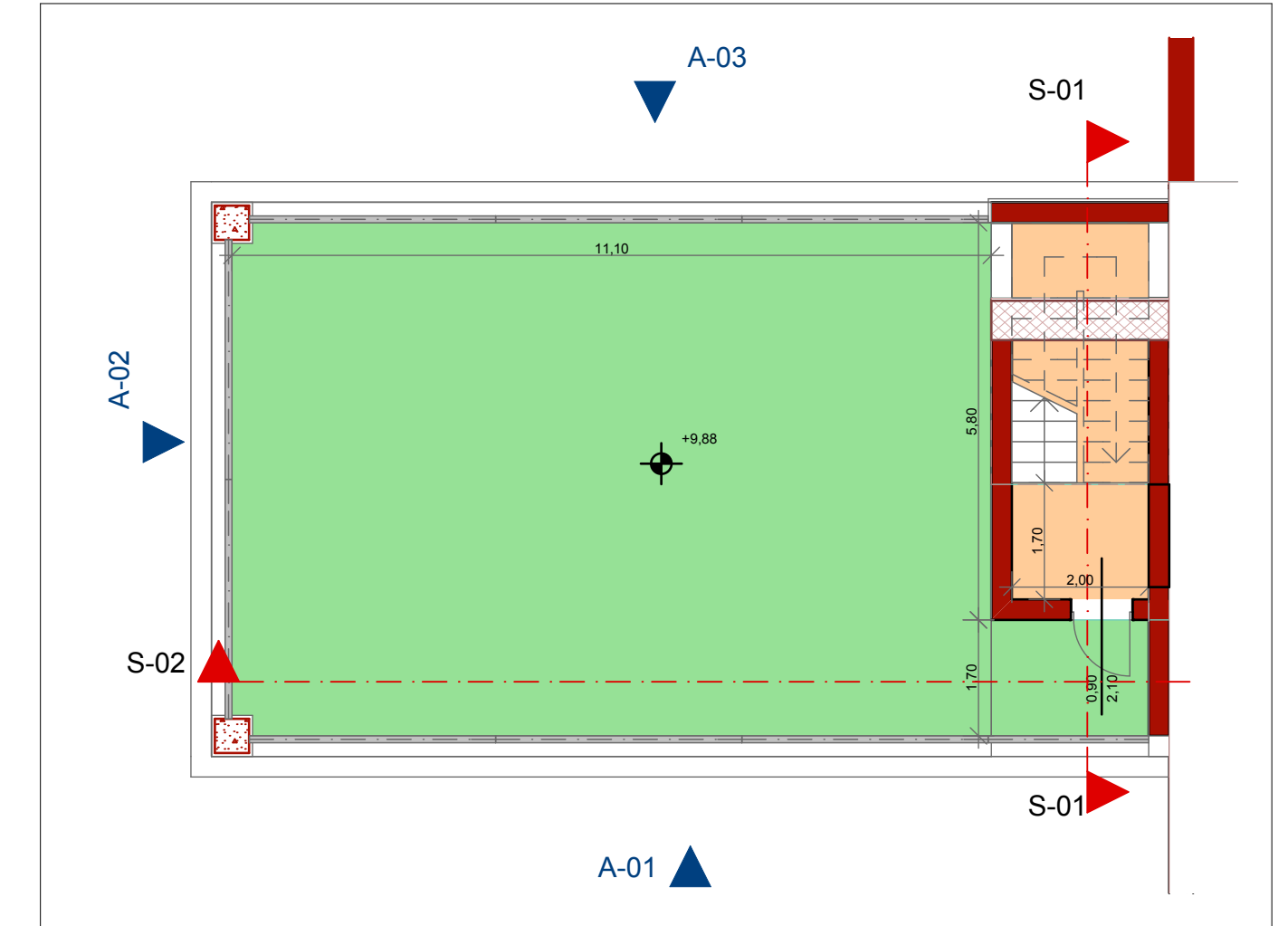
3. PIANO TERZO 1:100
