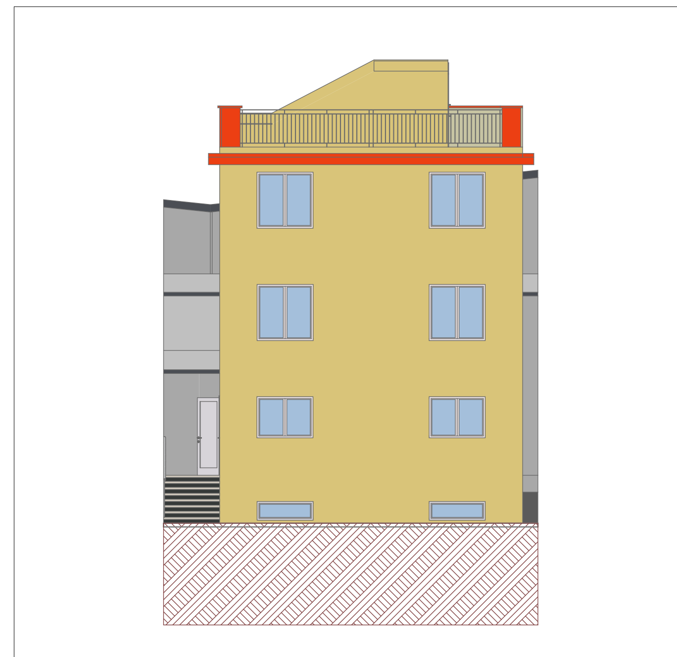
A-02 PROSPETTO 1:100
