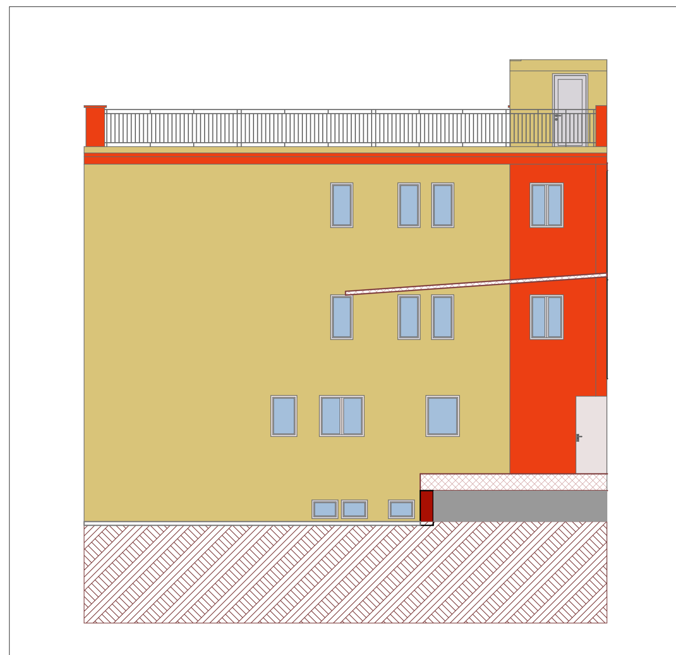
A-01 PROSPETTO 1:100
