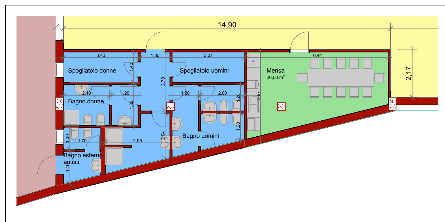
Particolare bagni 1:100
