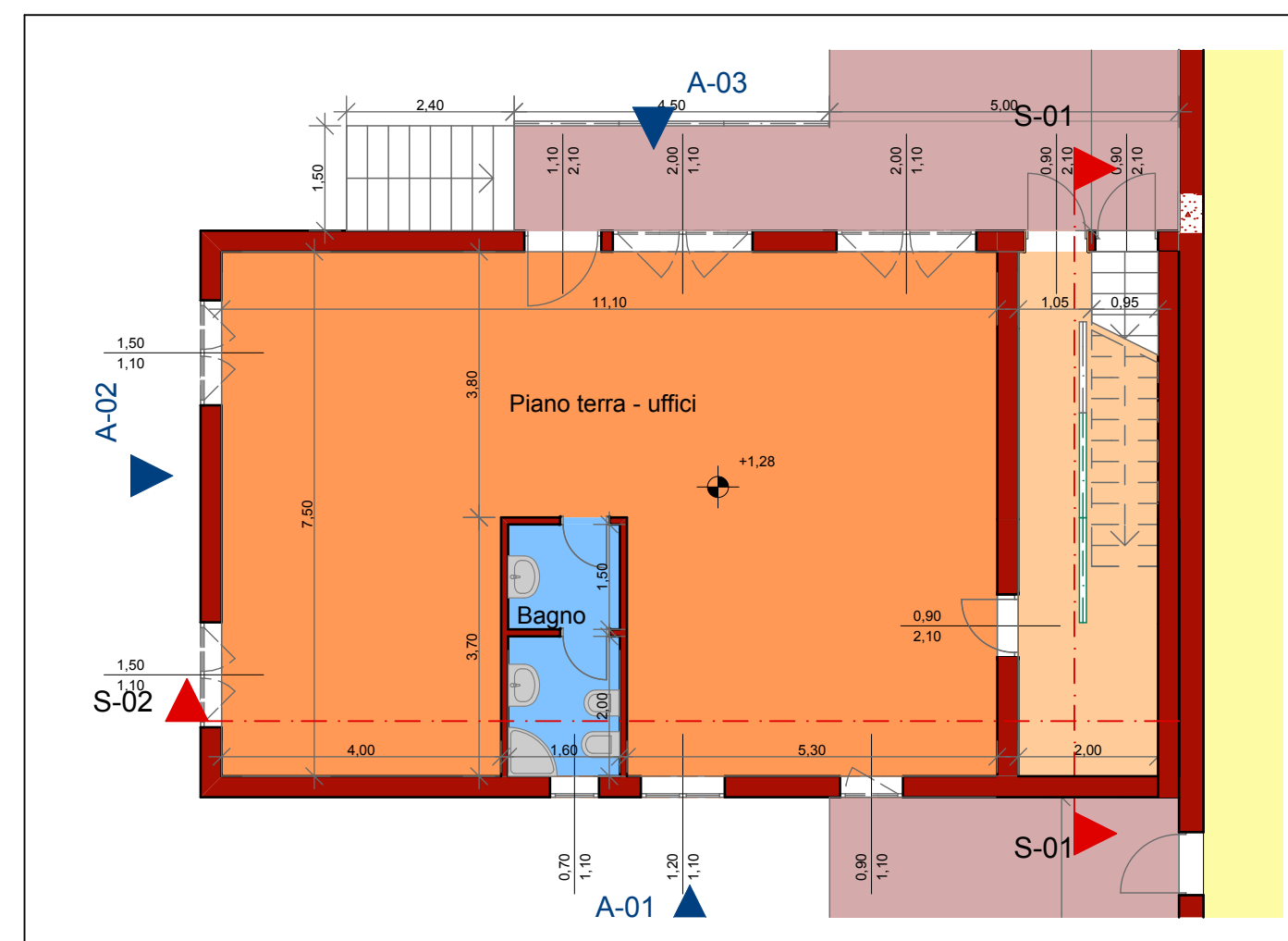
Particolare palazzina uffici - piano terra 1:100
