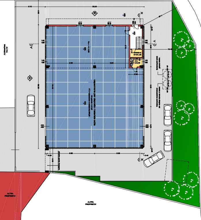
PIANTA PIANO TERZA - In Verifica (rapp. 1:100)
